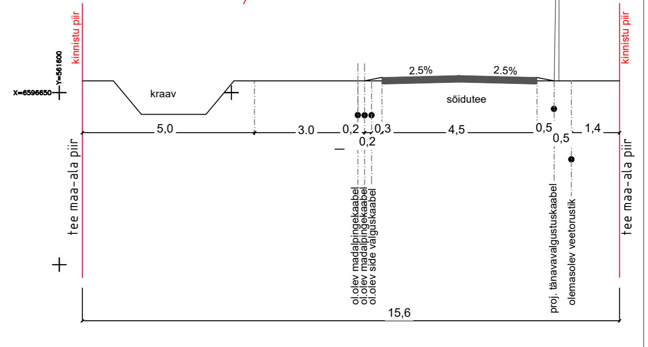
LÕIGE A-A M 1:100
