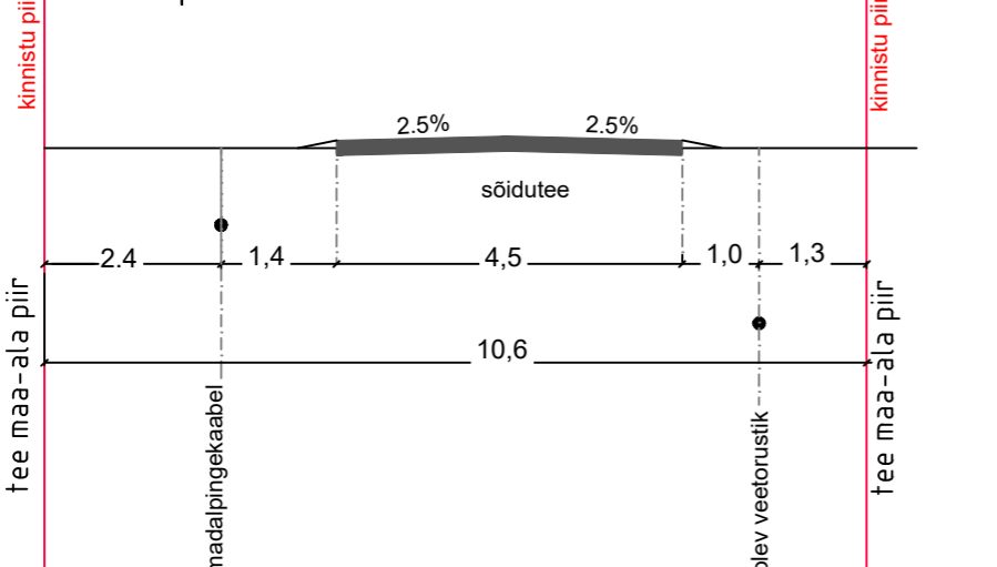
LÕIGE B-B M 1:100
